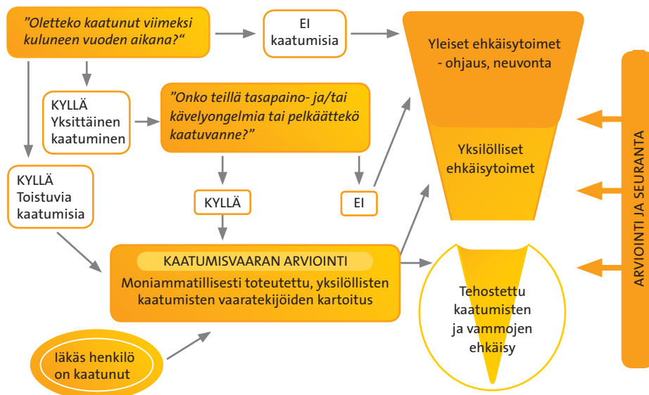
Kuvio 9. IKINÄ-malli.
